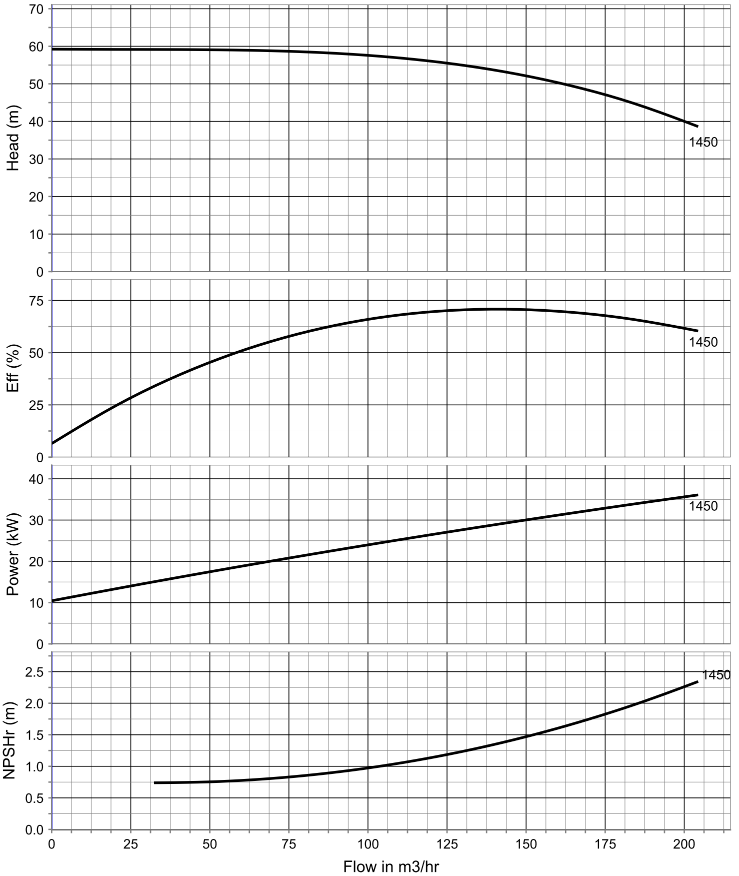
Impeller Dia : 409.0 mm , Stage : 1
