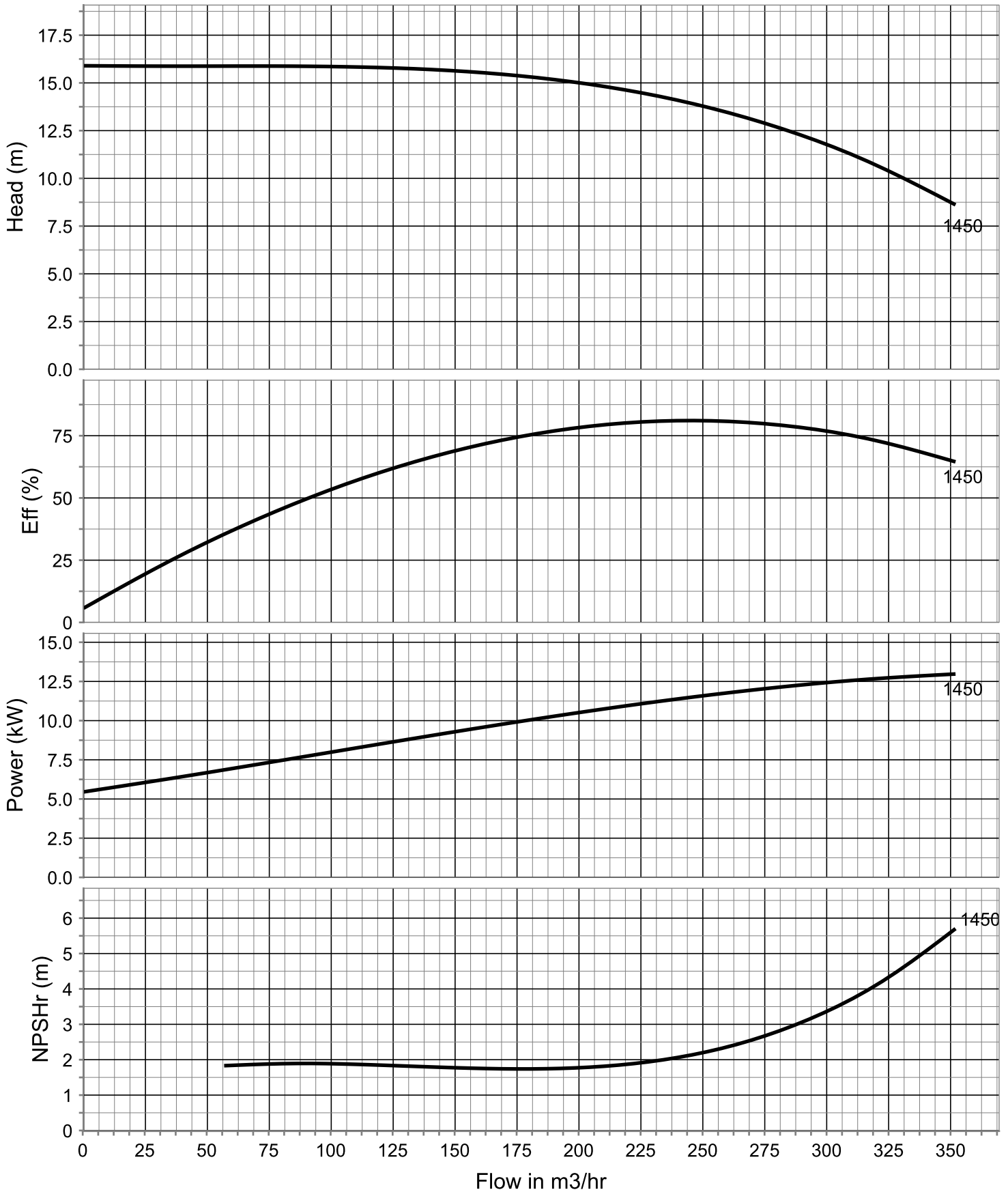
Impeller Dia : 220.0 mm , Stage : 1
